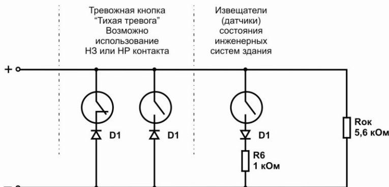
Рис.6. Схемы электрические принципиальные двух вариантов подключения охранного ШС.
