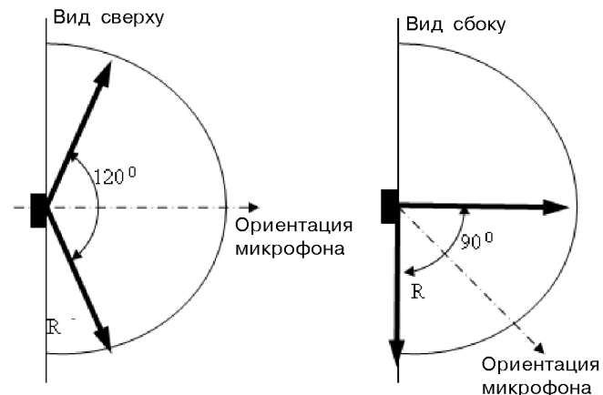
Рис. 1- Диаграмма зоны обнаружения АК-канала
