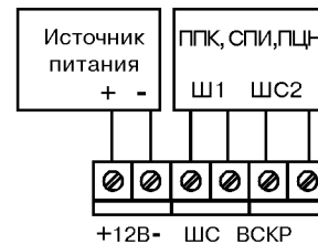
Рис. 2- Схема подключения извещателя с отдельными шлейфами сигнализации и вскрытия корпуса
