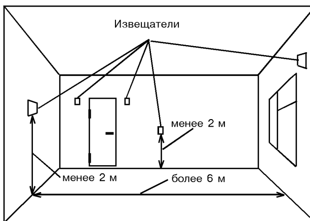
Рис. 9 - Не рекомендуемые места установки извещателя
