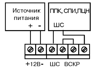
Рис. 3 - Схема подключения извещателя с объединенными шлейфами сигнализации и вскрытия корпуса
